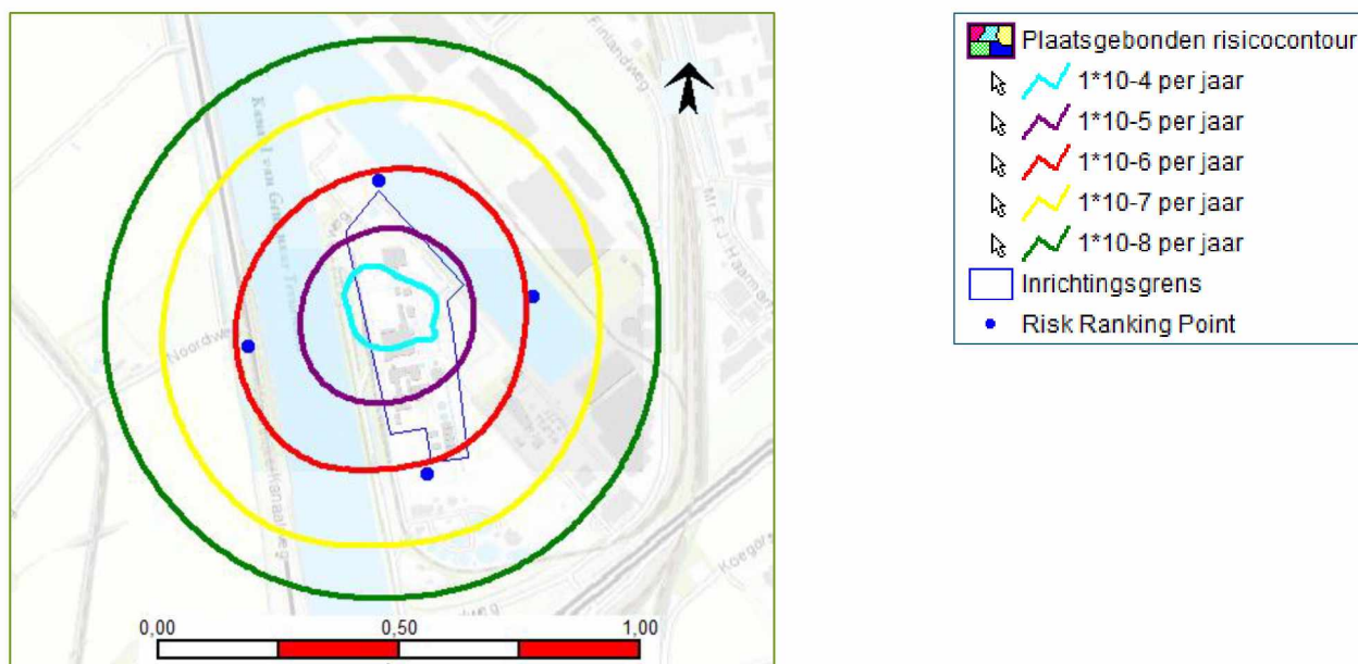
Figuur 4.4. Plaatsgebonden risicocontouren Safeti-NL versie 8.21 [5]
