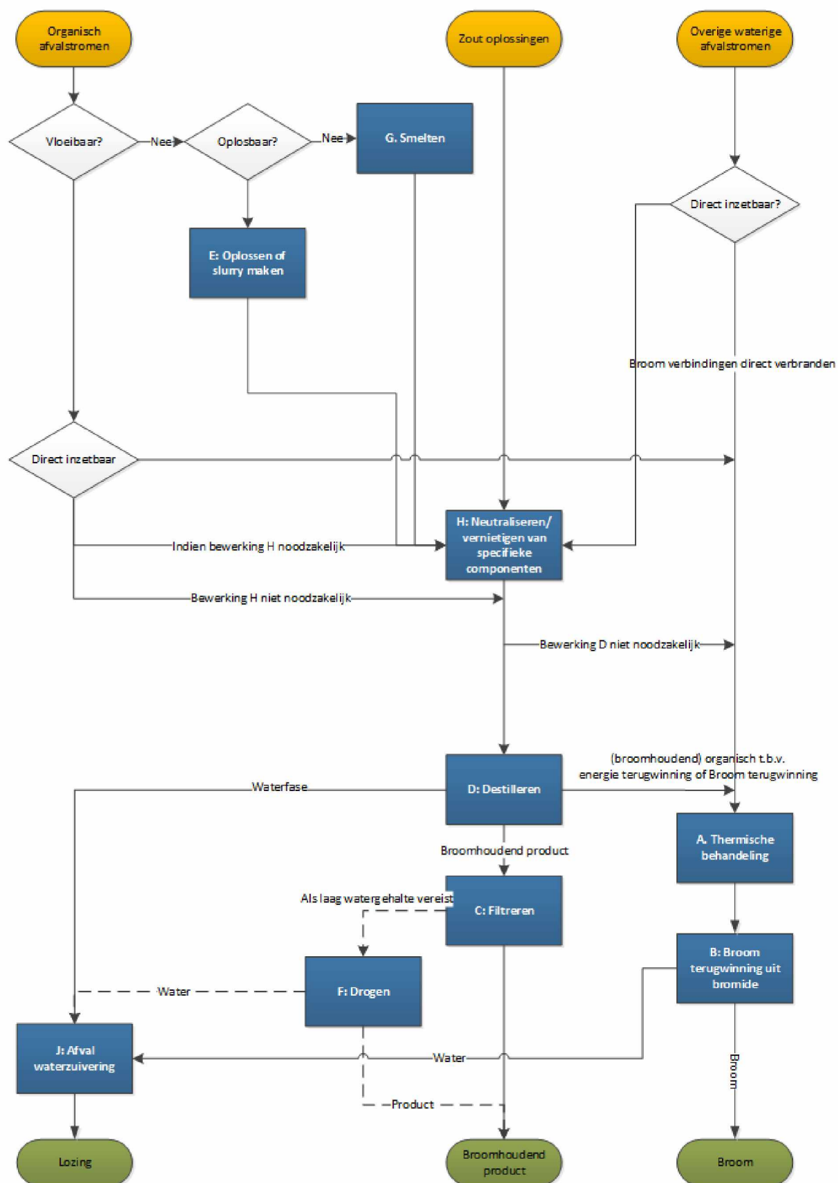
Figuur 1: Stroomschema van afvalverwerkingsroutes ICL-IP
