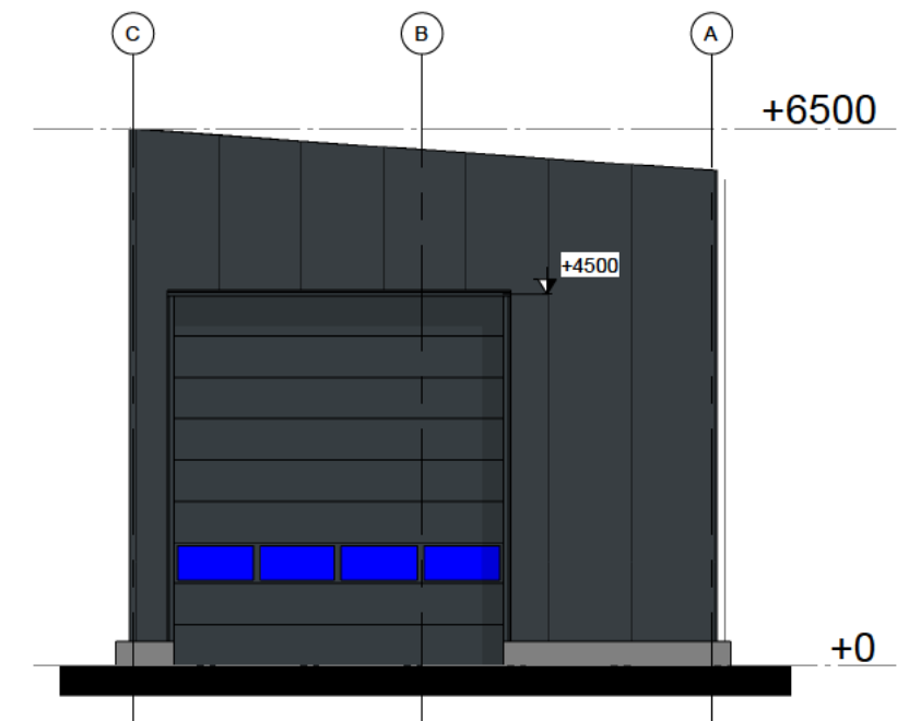
Achtergevel
