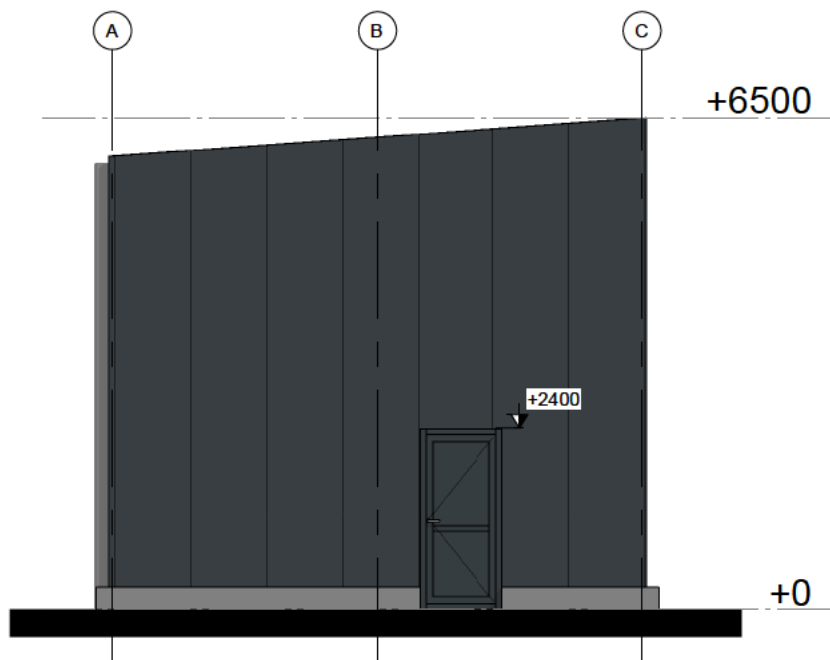
Voorgevel
