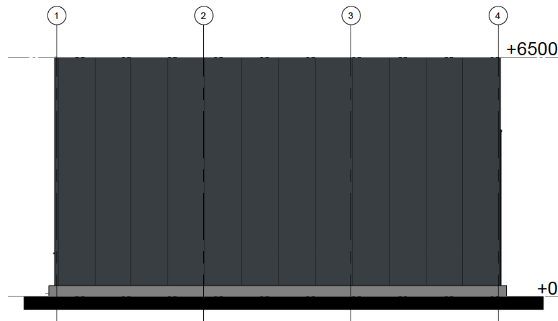
Rechtergevel
