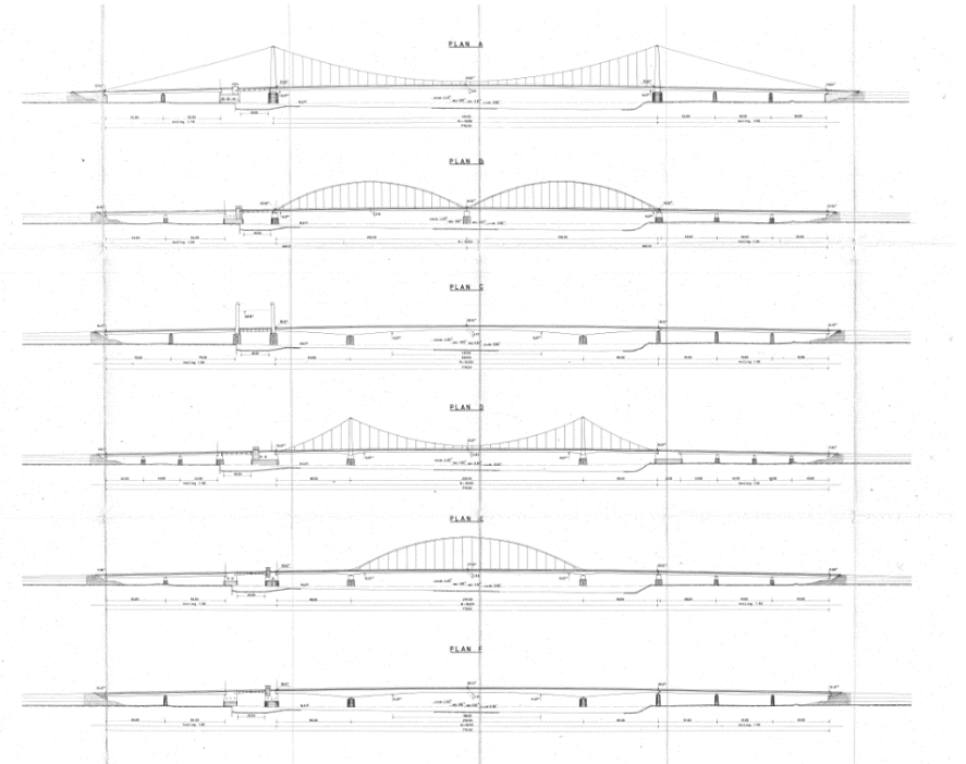
Overzicht van de verschillende plannen voor de Merwedebrug. Uiteindelijk is gekozen voor plan B. RWS bouwdoos C 427A, nr. C7464.
