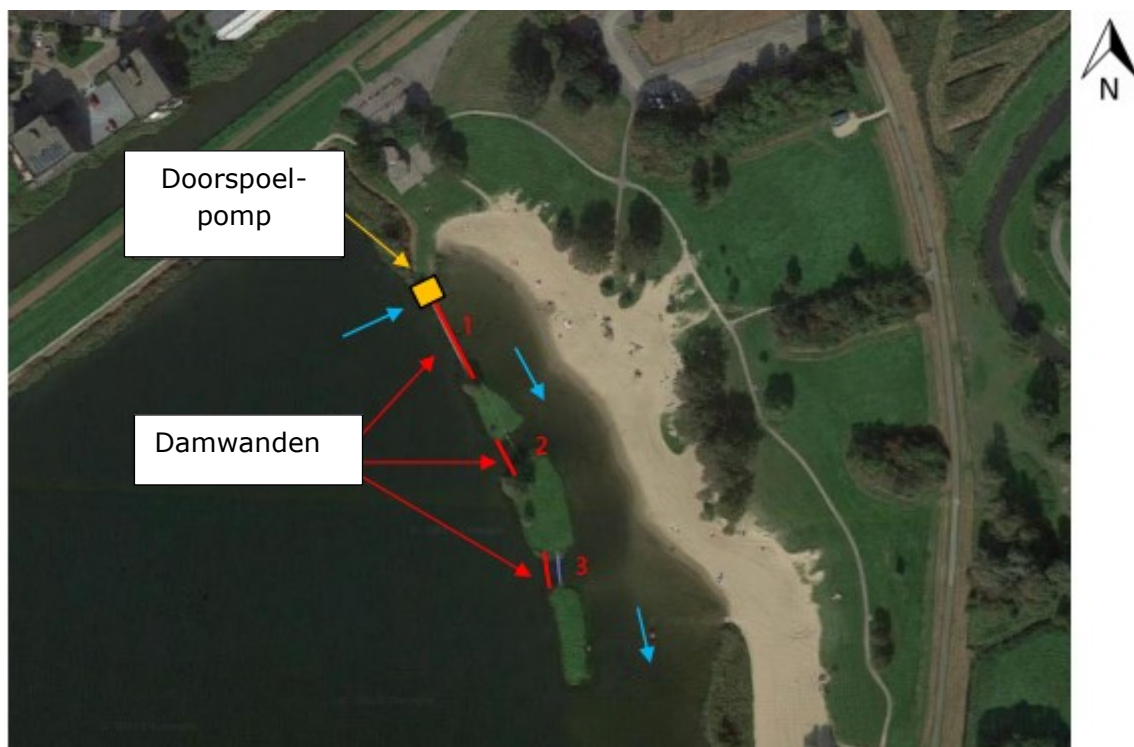
Figuur 2.2 Toekomstige situatie met doorspoelbaar zwemcompartiment
