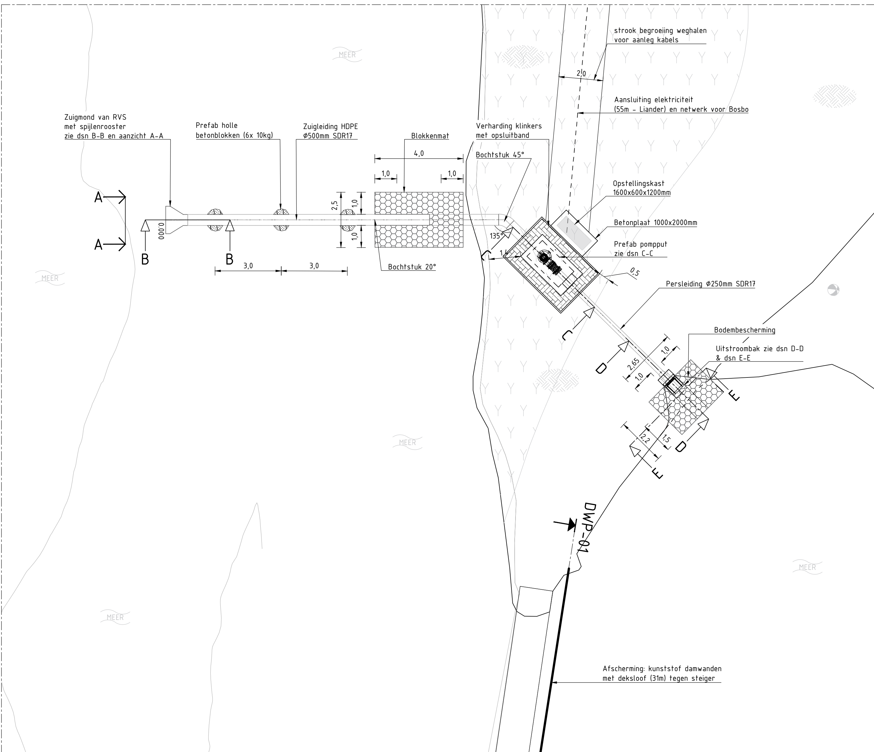
BOVENAANZICHT MECHANISCHE DOORSPOELING Schaal 1:100
