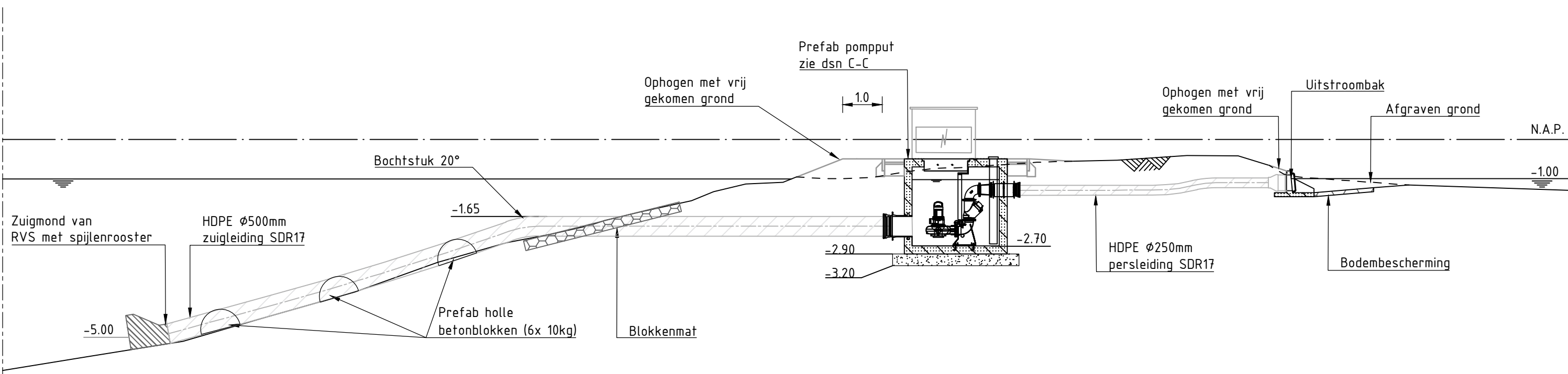
ZIJDEAANZICHT MECHANISCHE DOORSPOELING Schaal 1:100
