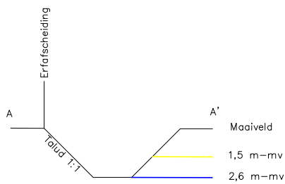
Dwarsdoorsnede geplande ontgraving
