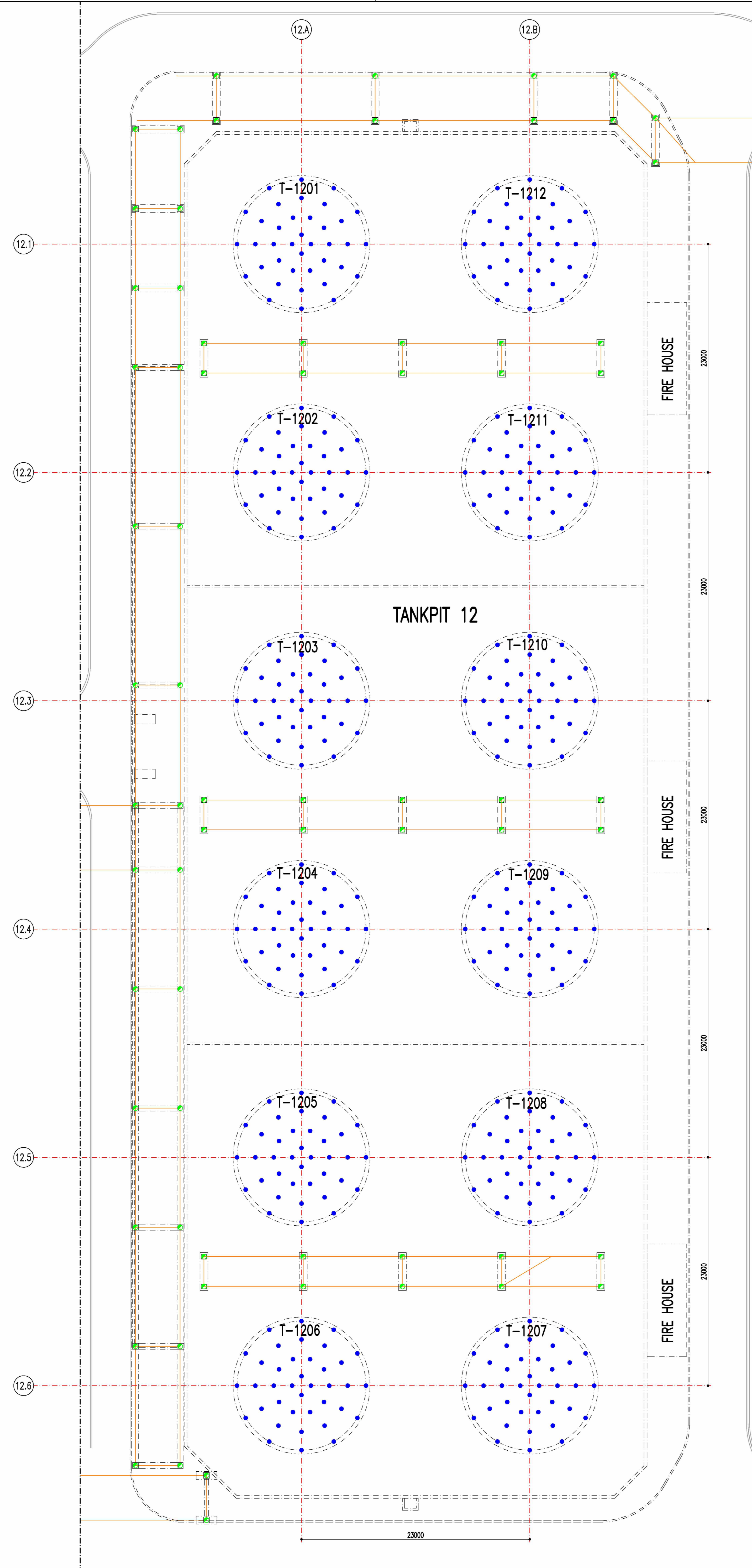
GRONDPLAN TANKPIT 12 SCHAL 1/200
