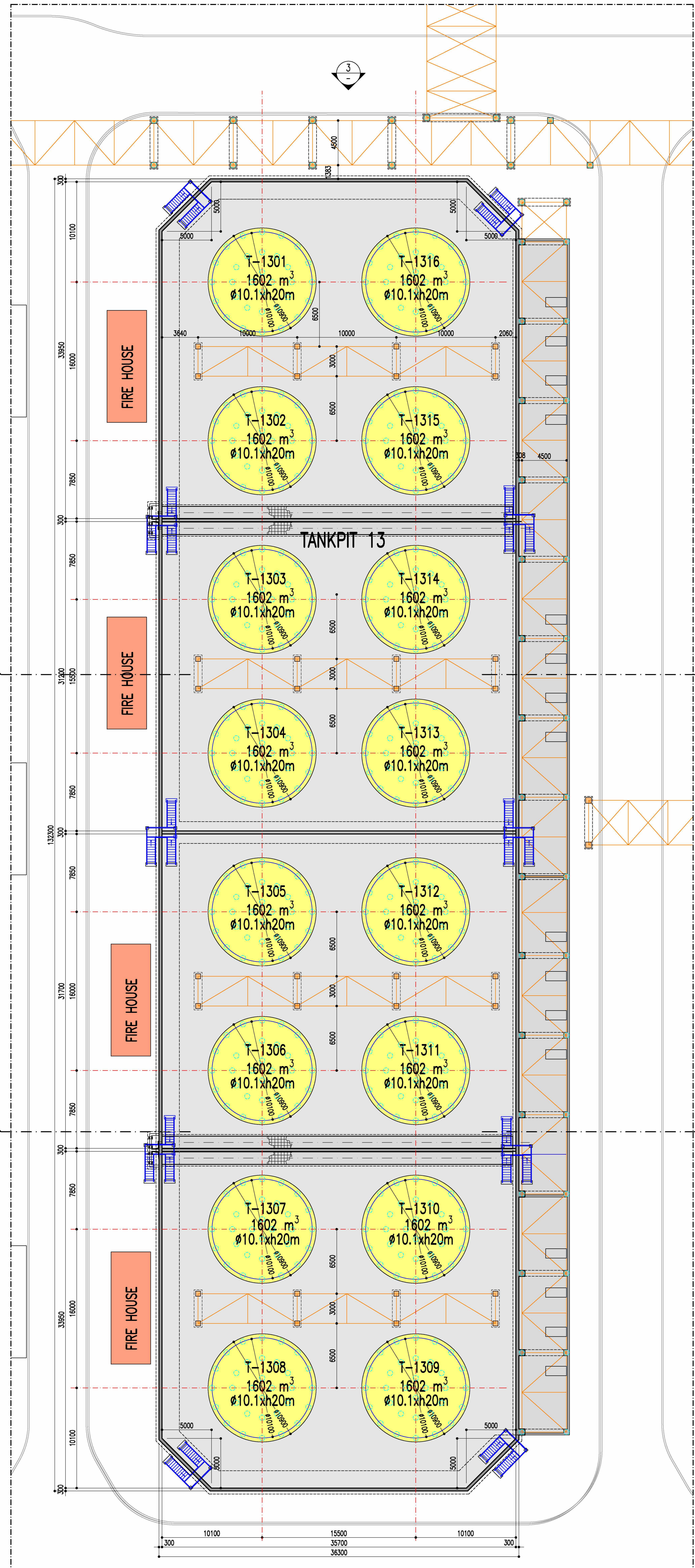
GRONDPLAN TANKPIT 13 SCHAL. 1/200
