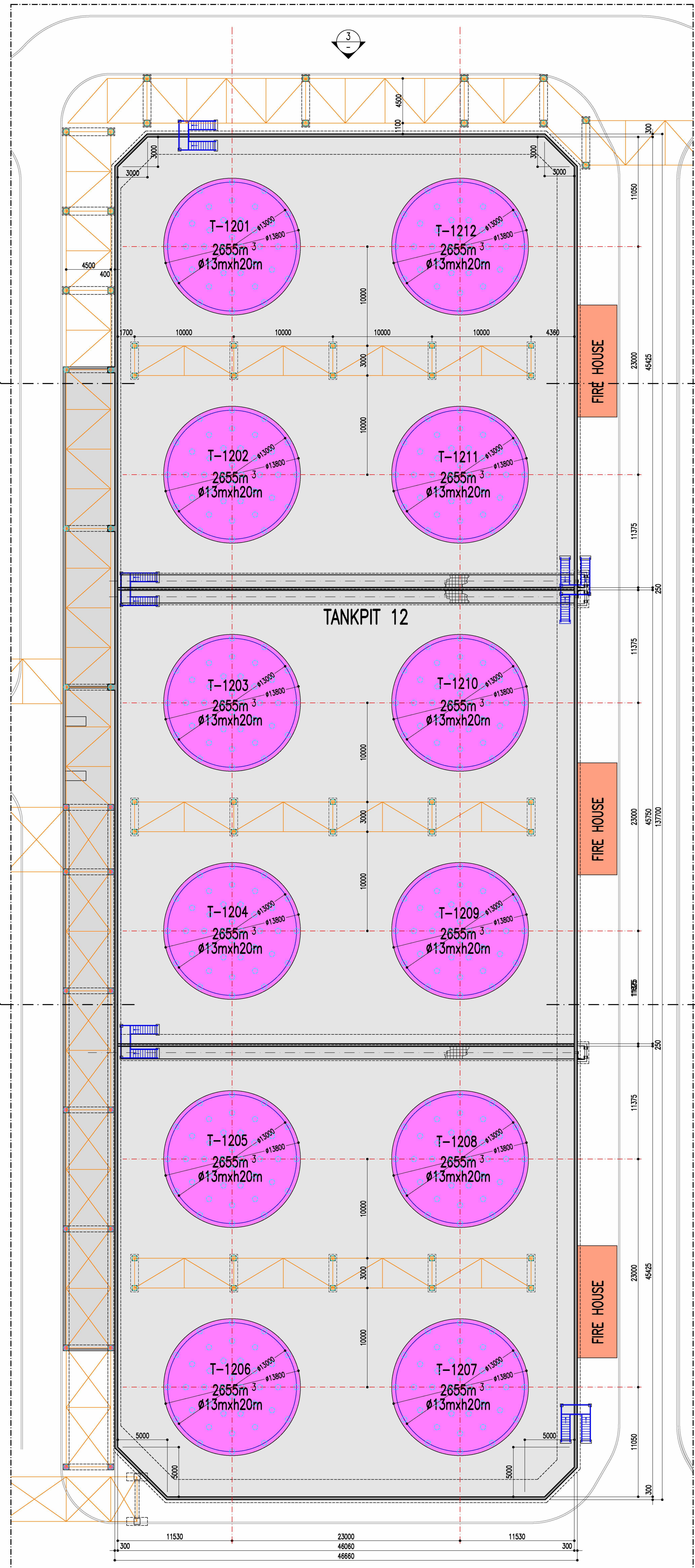
GRONDPLAN TANKPIT 12 SCHAL 1/200
