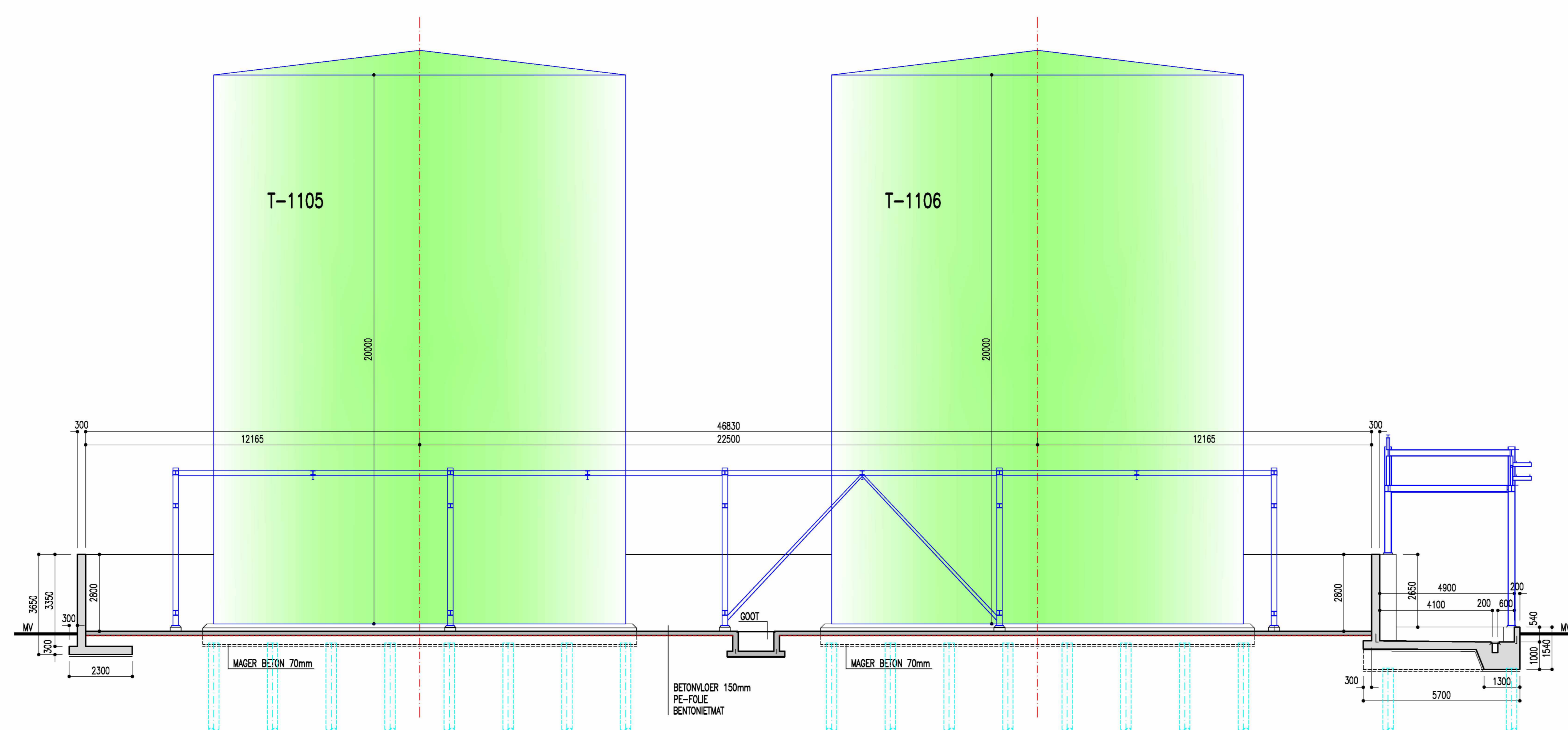
DOORSNEDE SCHAAL 1/100
