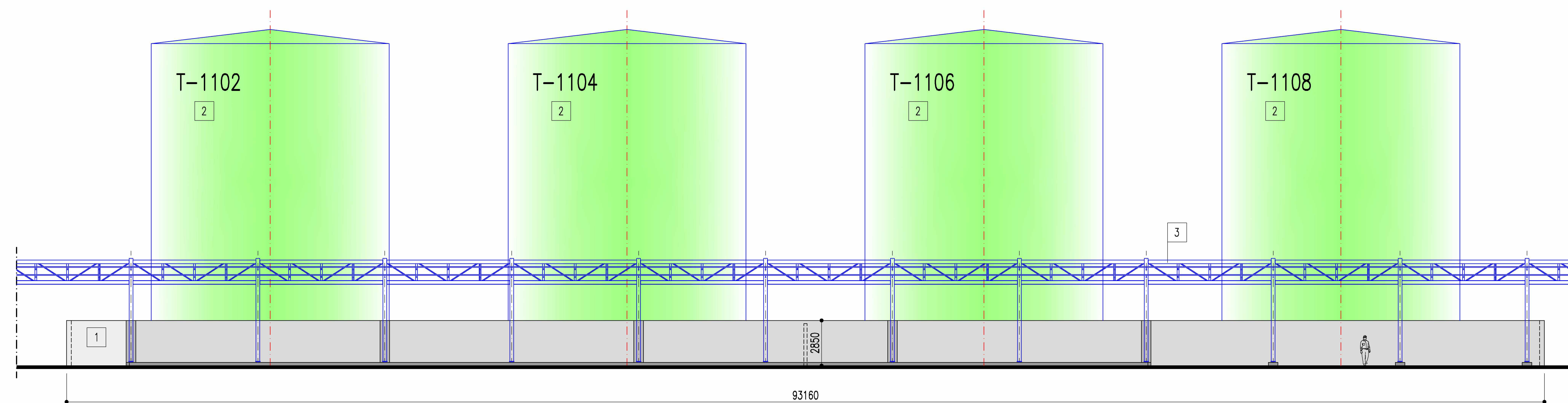
1 GEVEL SCHAAL 1/200
