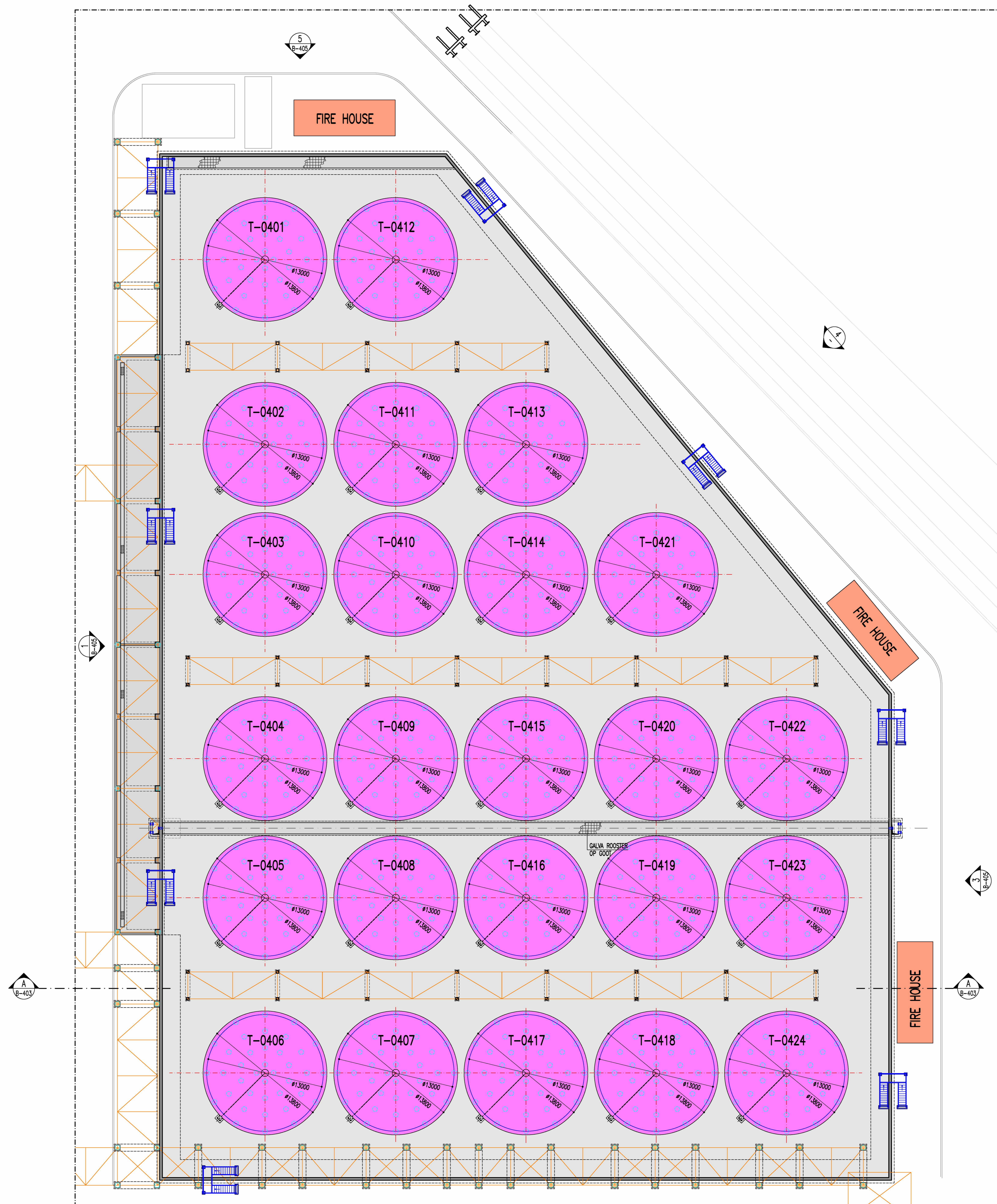
GRONDPLAN SCHAL. 1/200
