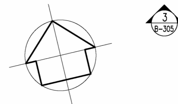
GRONDPLAN TANKPIT 3 SCHAL 1/200
