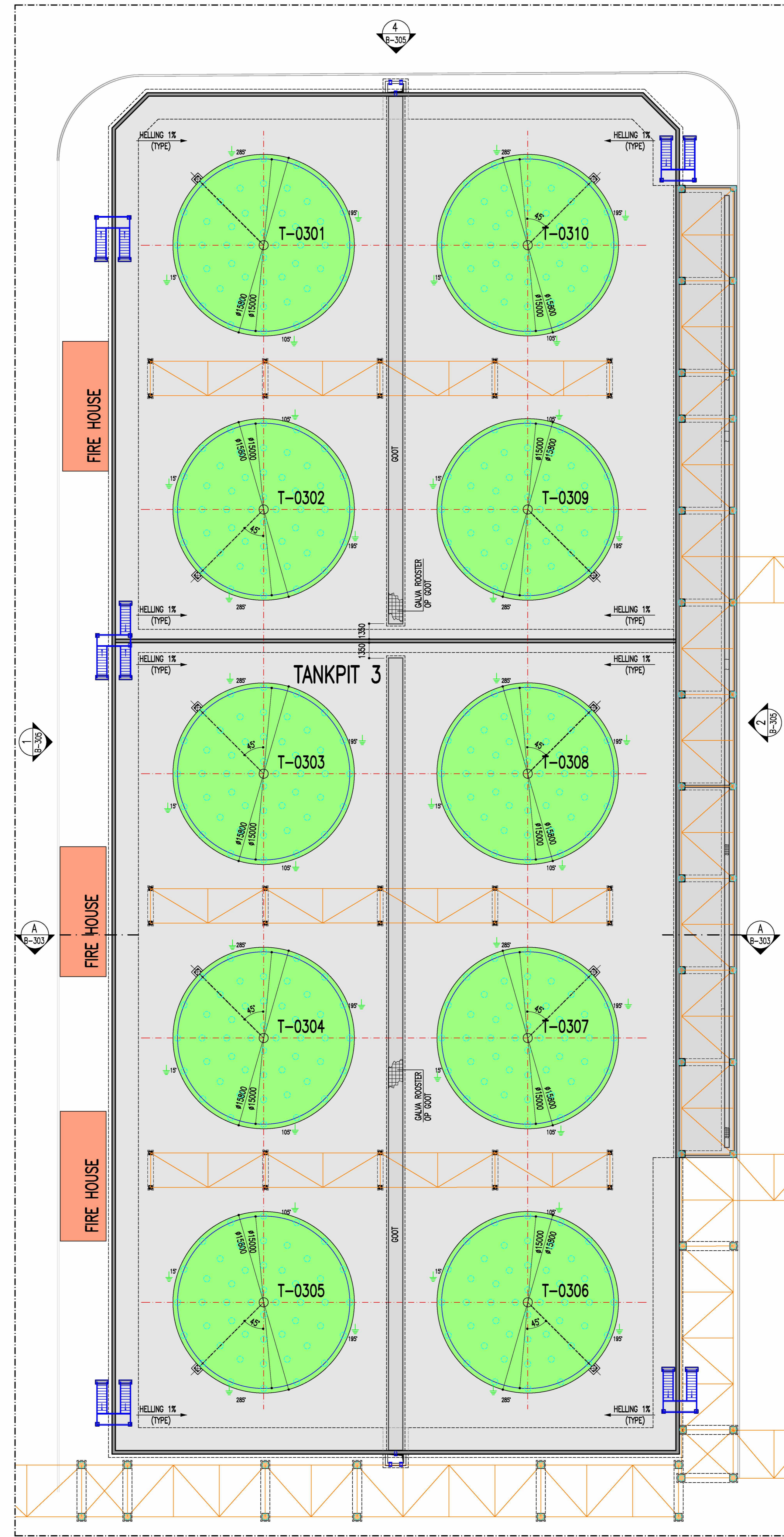
GRONDPLAN TANKPIT 3 SCHAL 1/200
