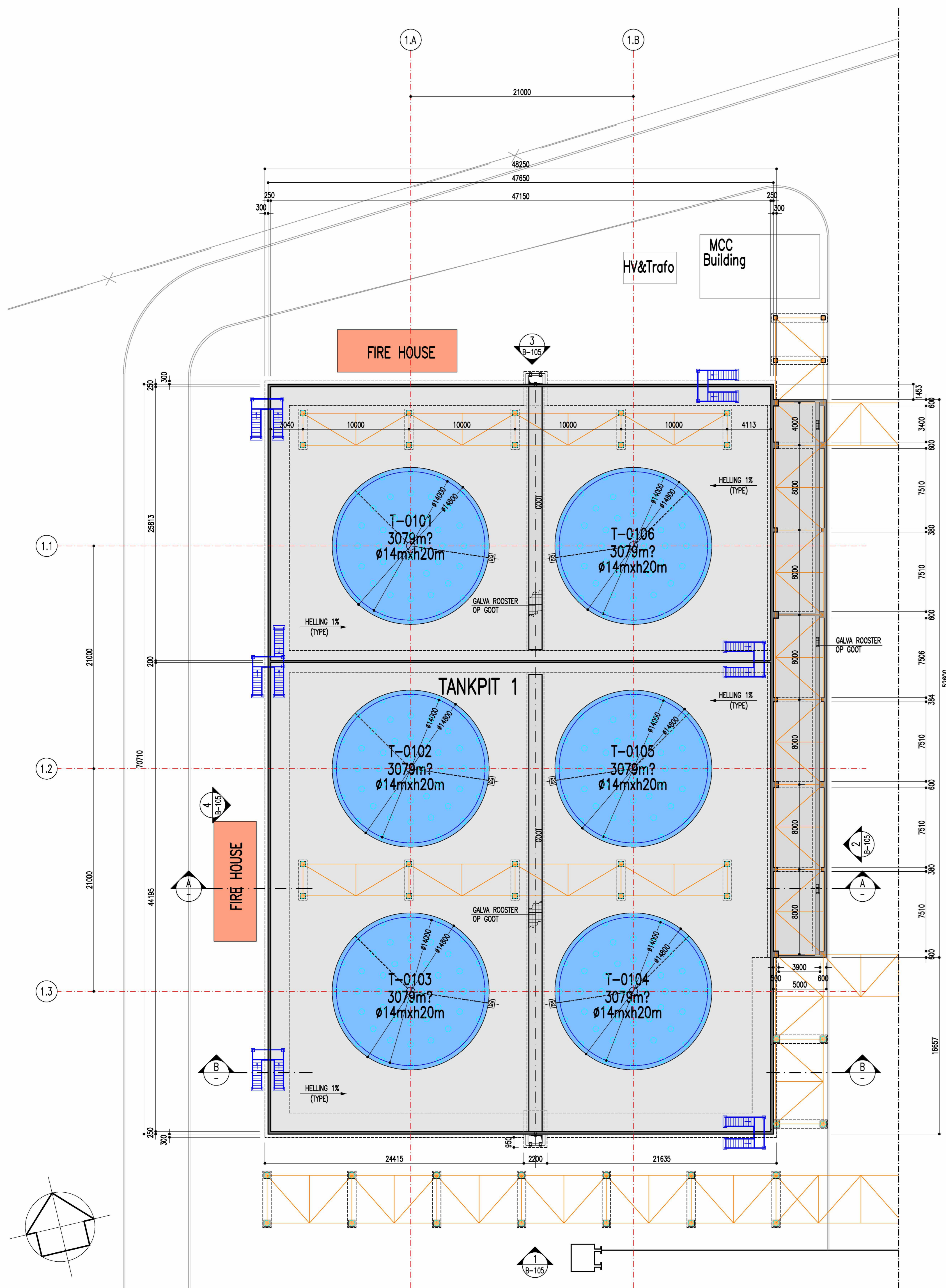
GRONDPLAN TANKPIT 1 SCHAL 1/200
