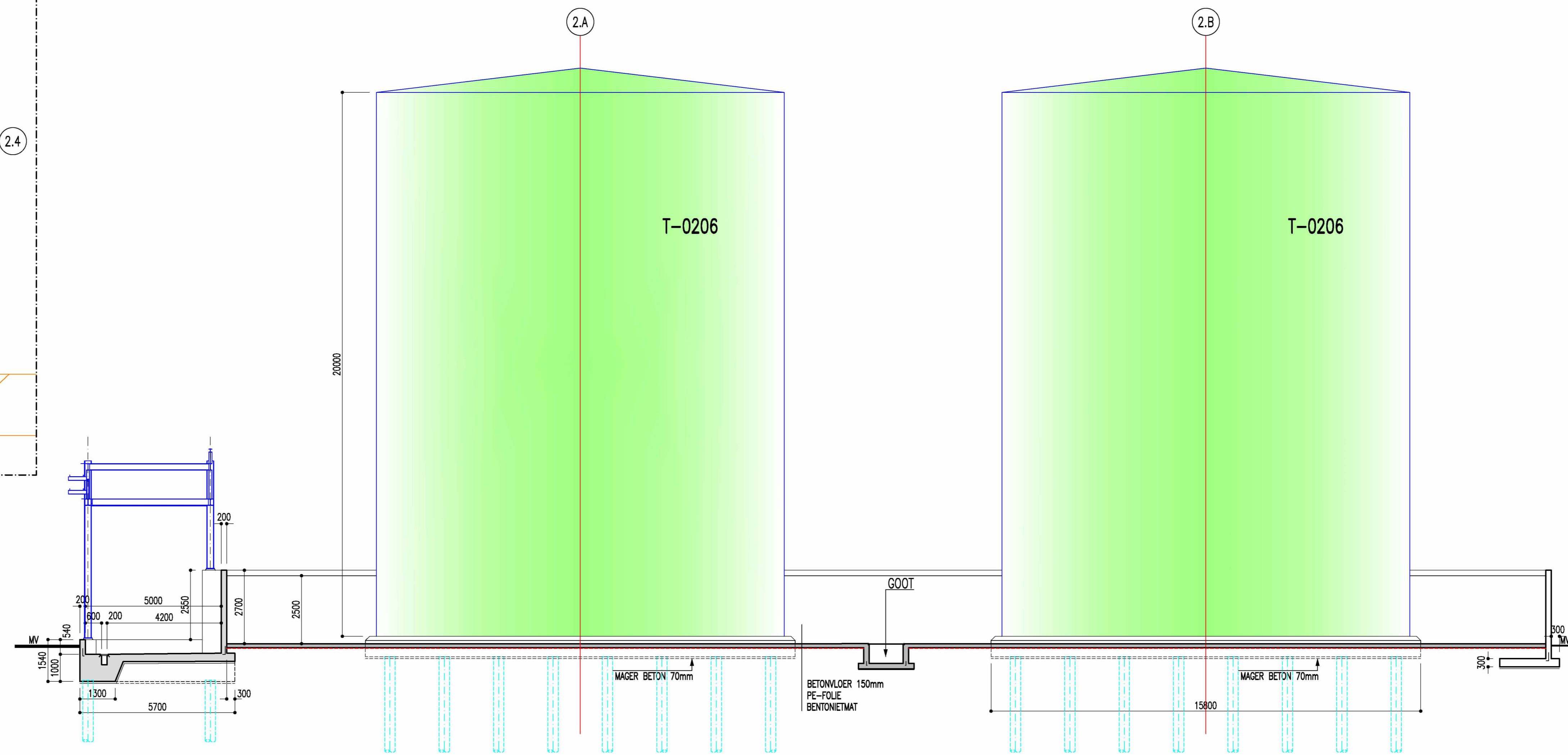
DOORSNEDE SCHAL. 1/100
