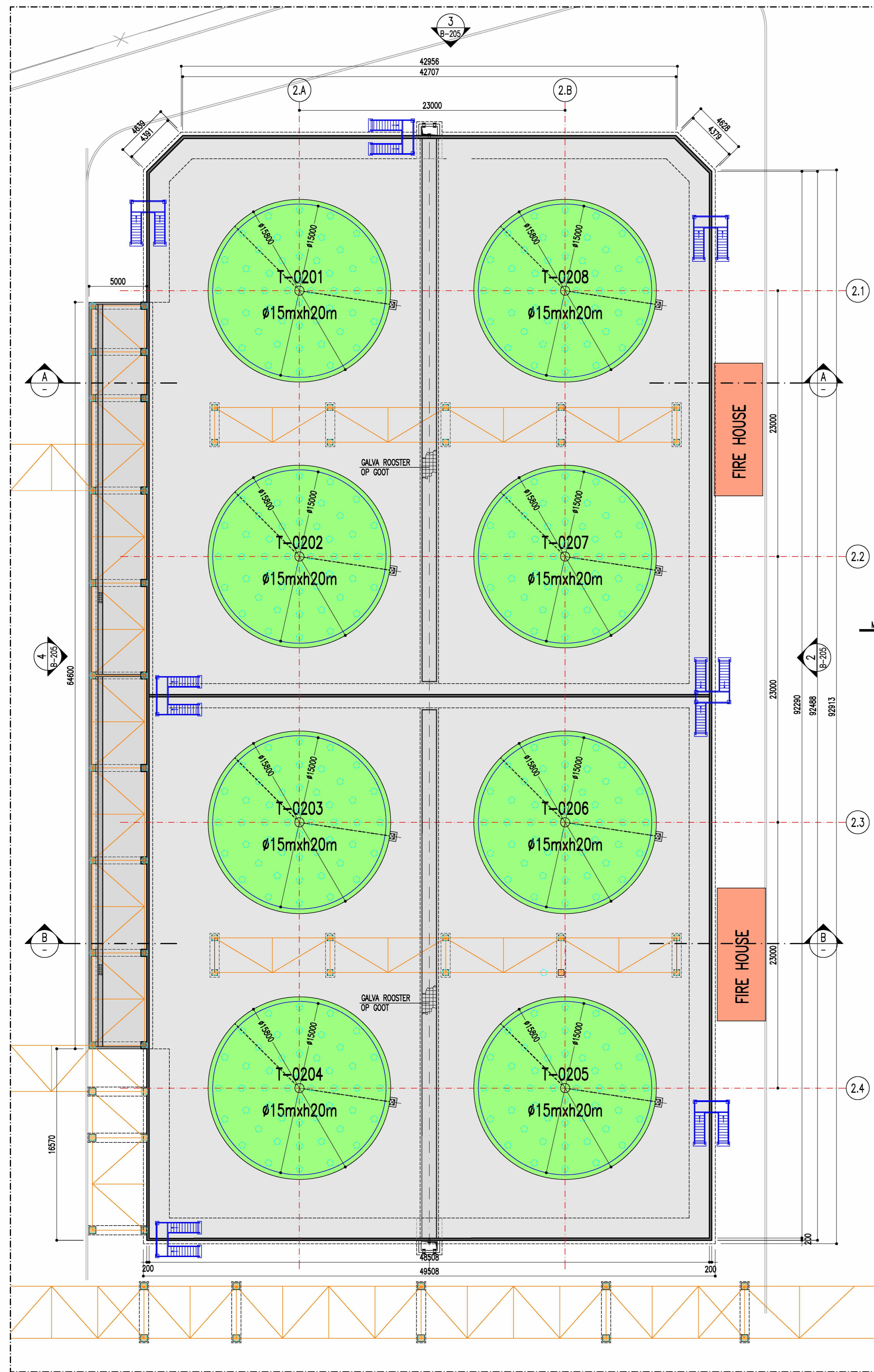
GRONDPLAN SCHAL. 1/200
