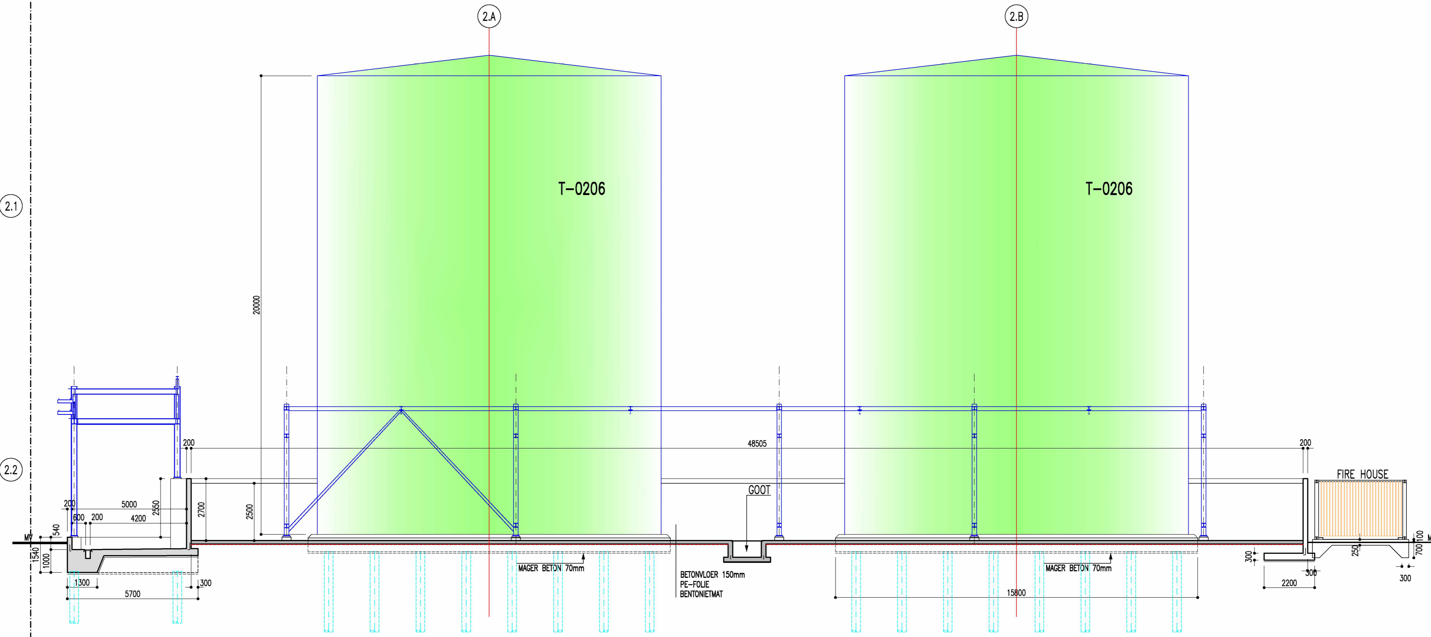
DOORSNEDE SCHAL. 1/100
