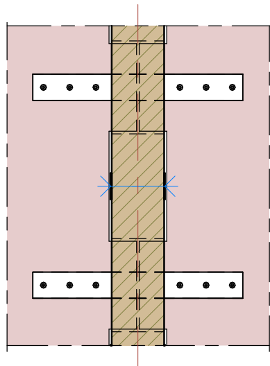
bovenaanzicht
