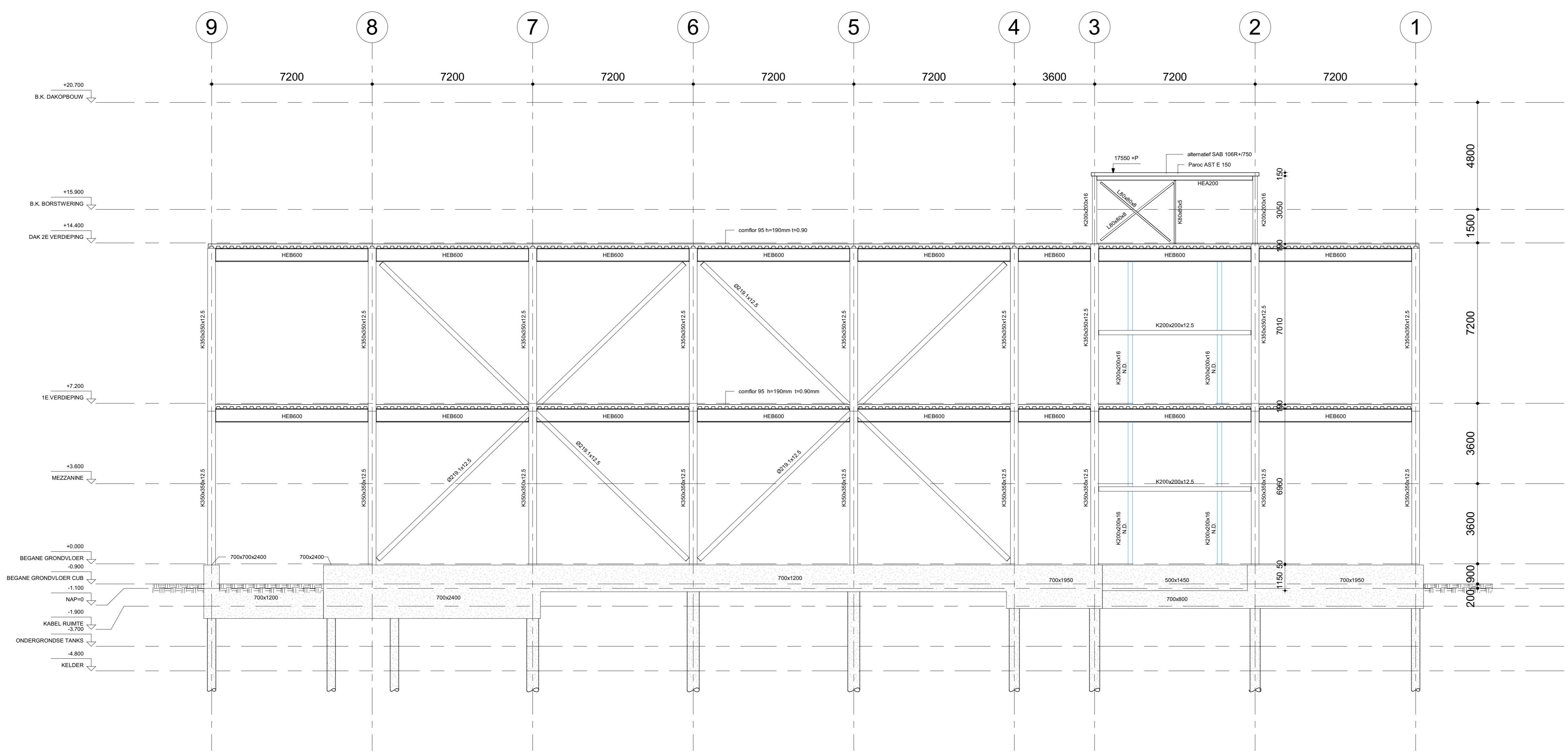
1 WESTGEVEL Schaal: 1:100
