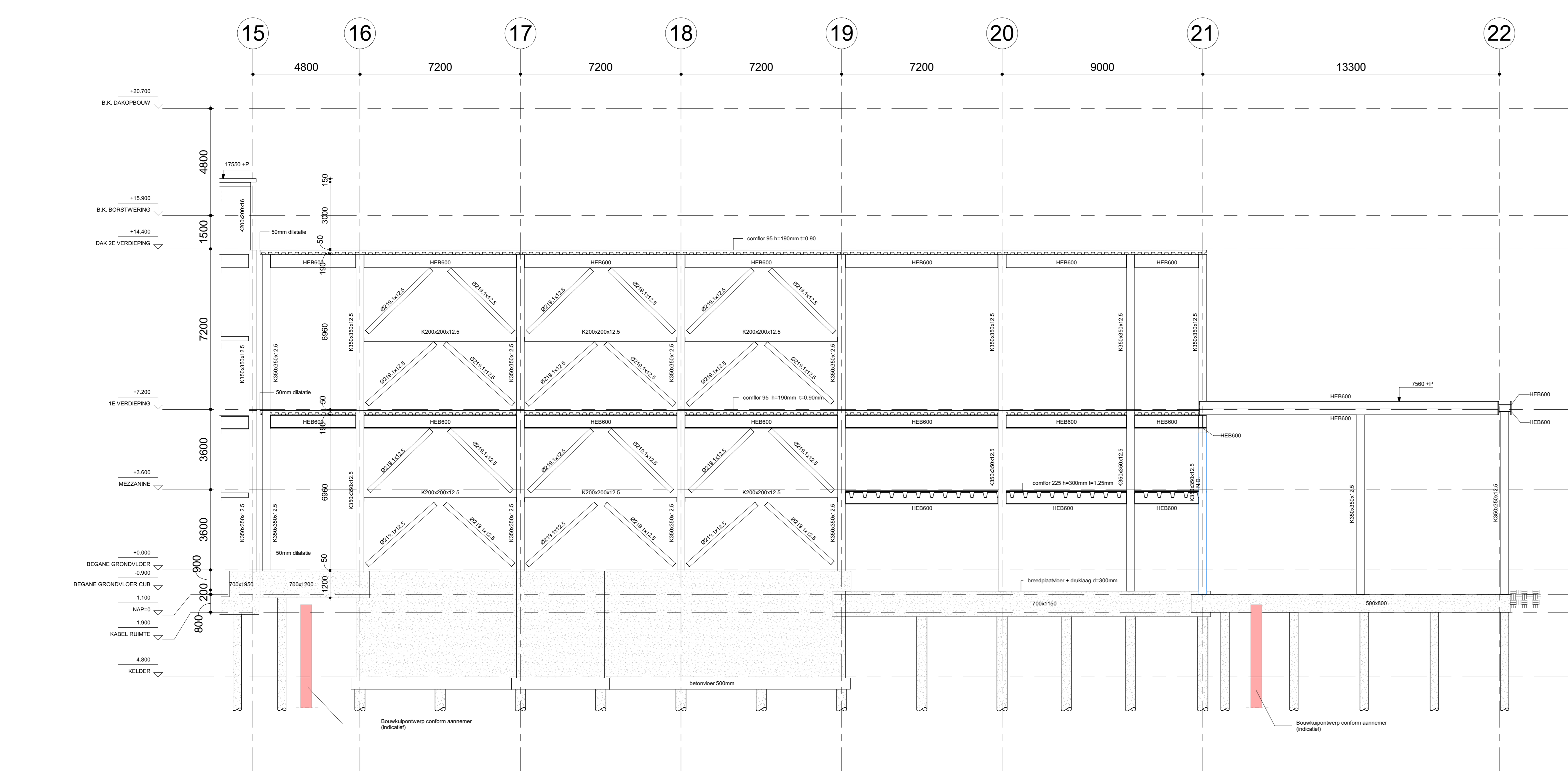
1 OOSTGEVEL Schaal: 1:100
