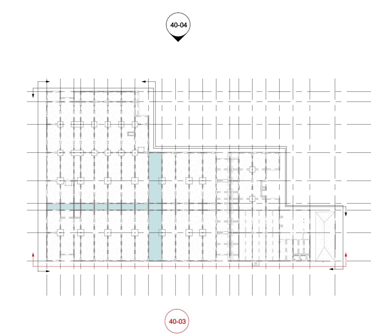
Situatie Schaal: 1:1000
