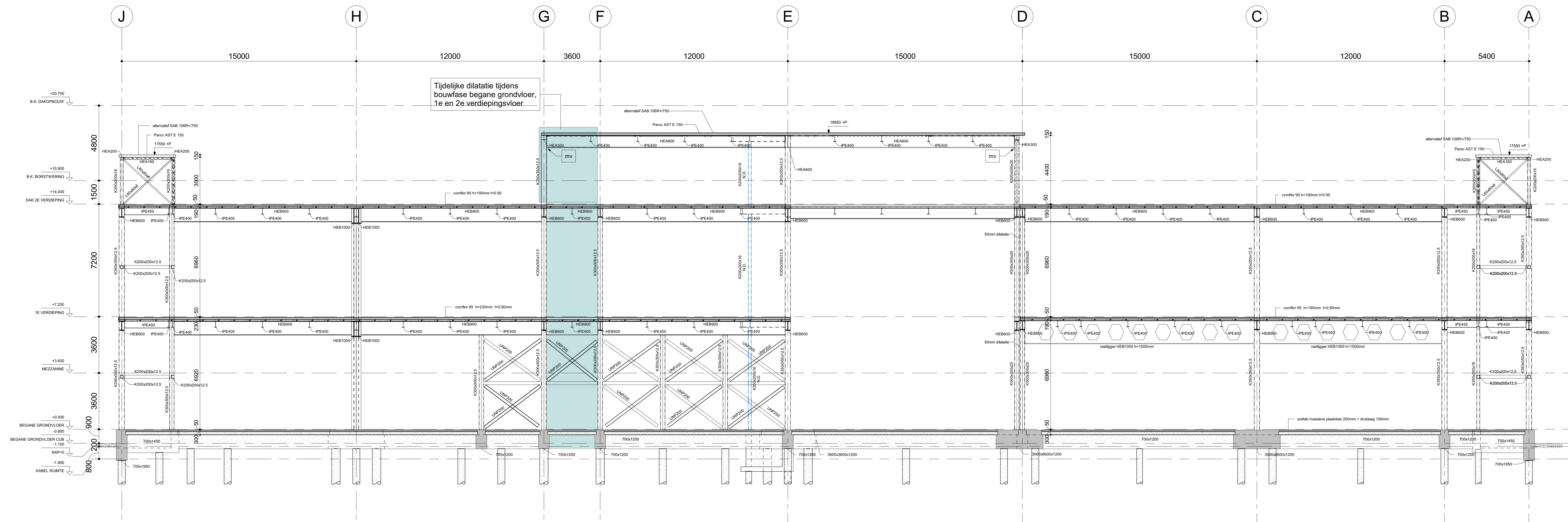
E DOORSNEDE Schaal: 1:100
