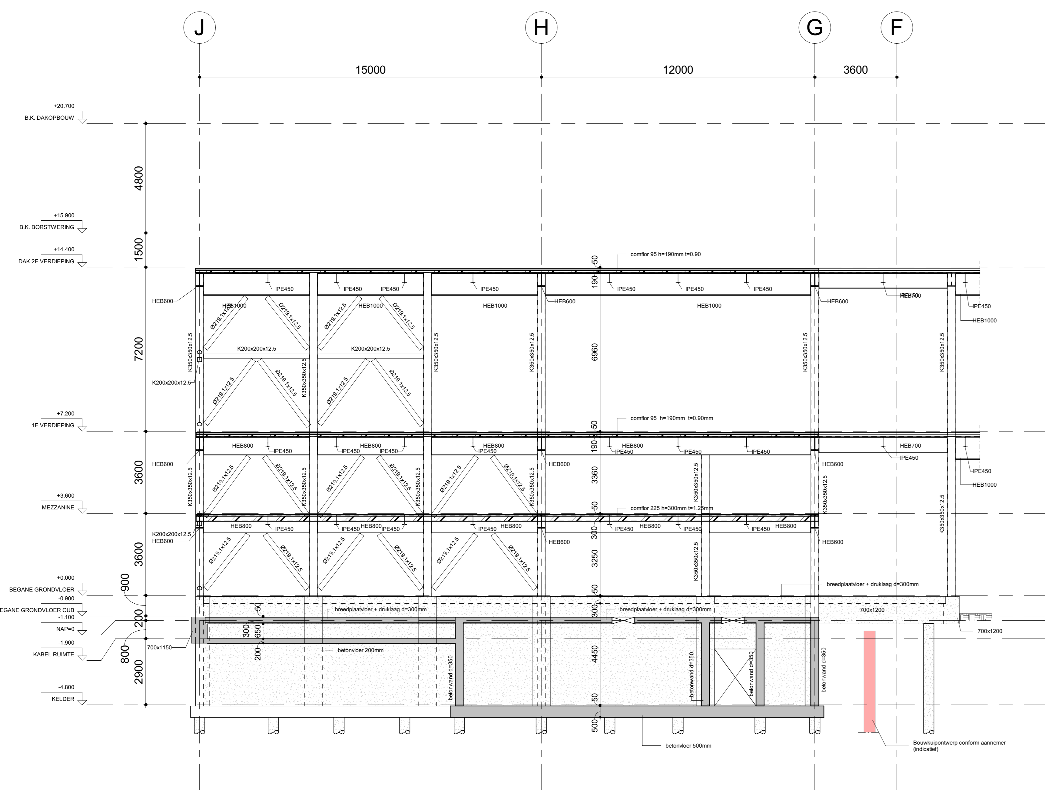
C DOORSNEDE Schaal: 1 : 100
