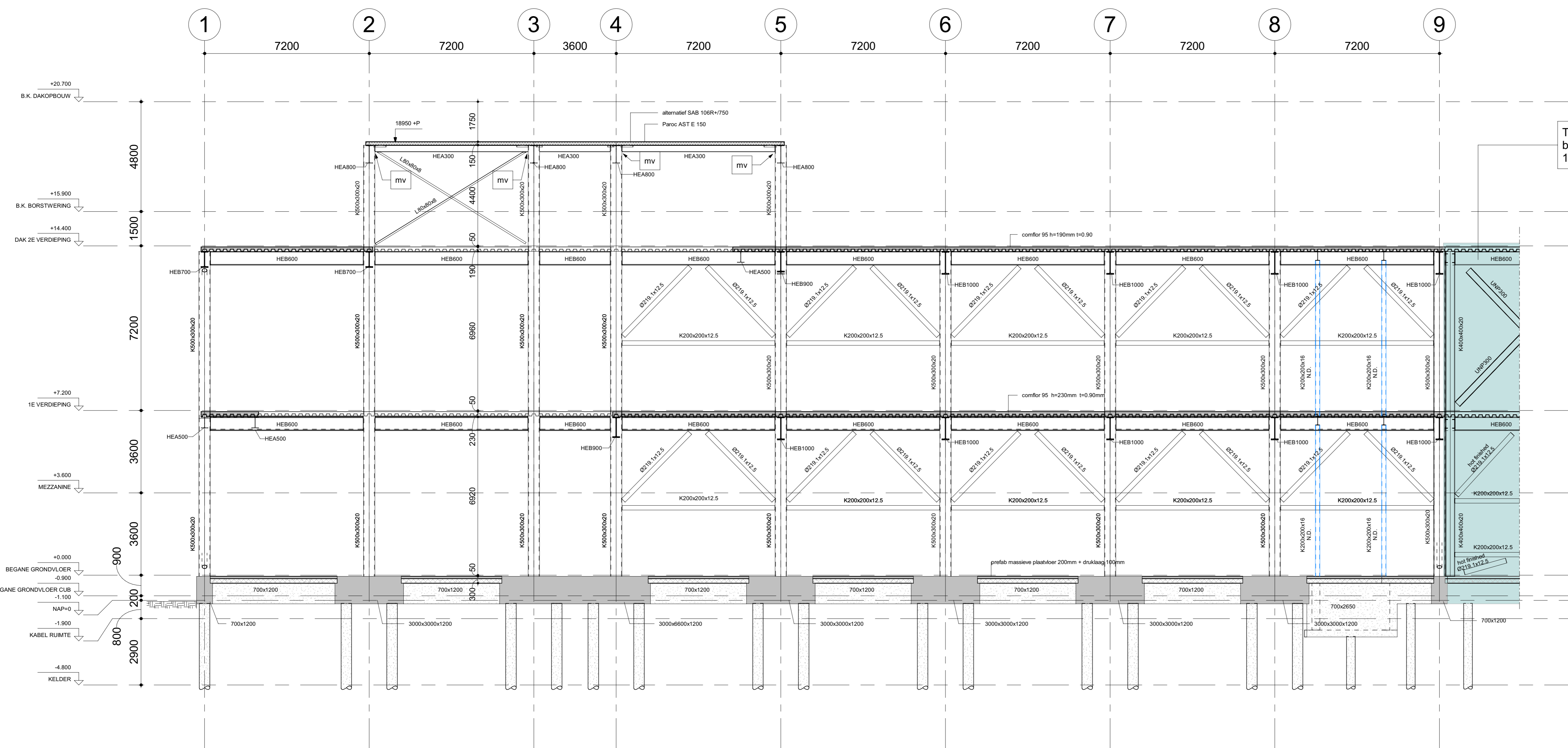
B DOORSNEDE Schaal: 1 : 100
