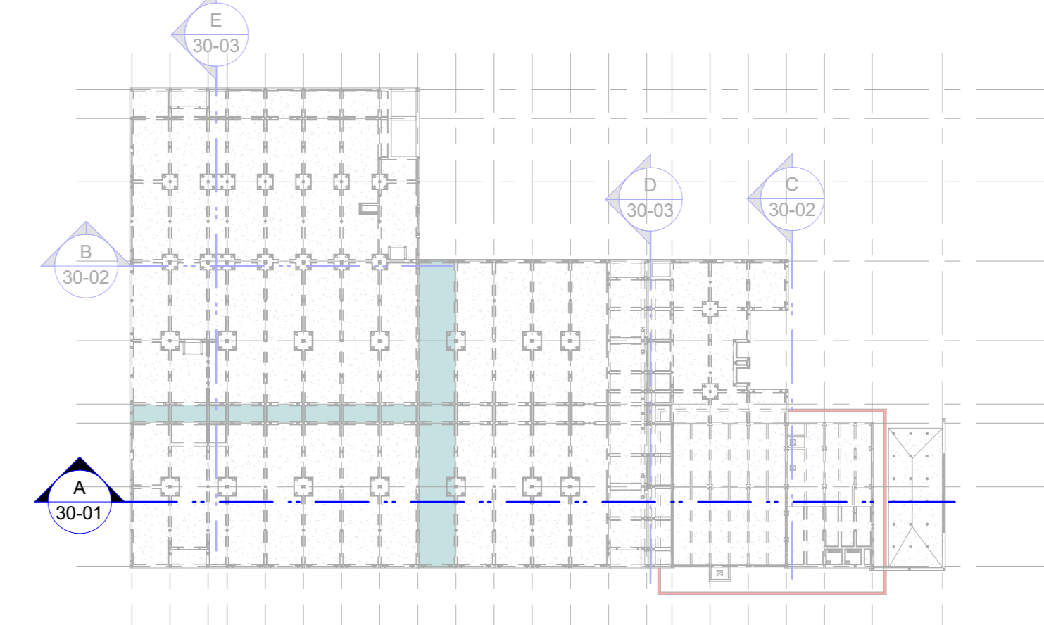
OVERZICHT DOORSNEDEN Schaal: 1:1000
