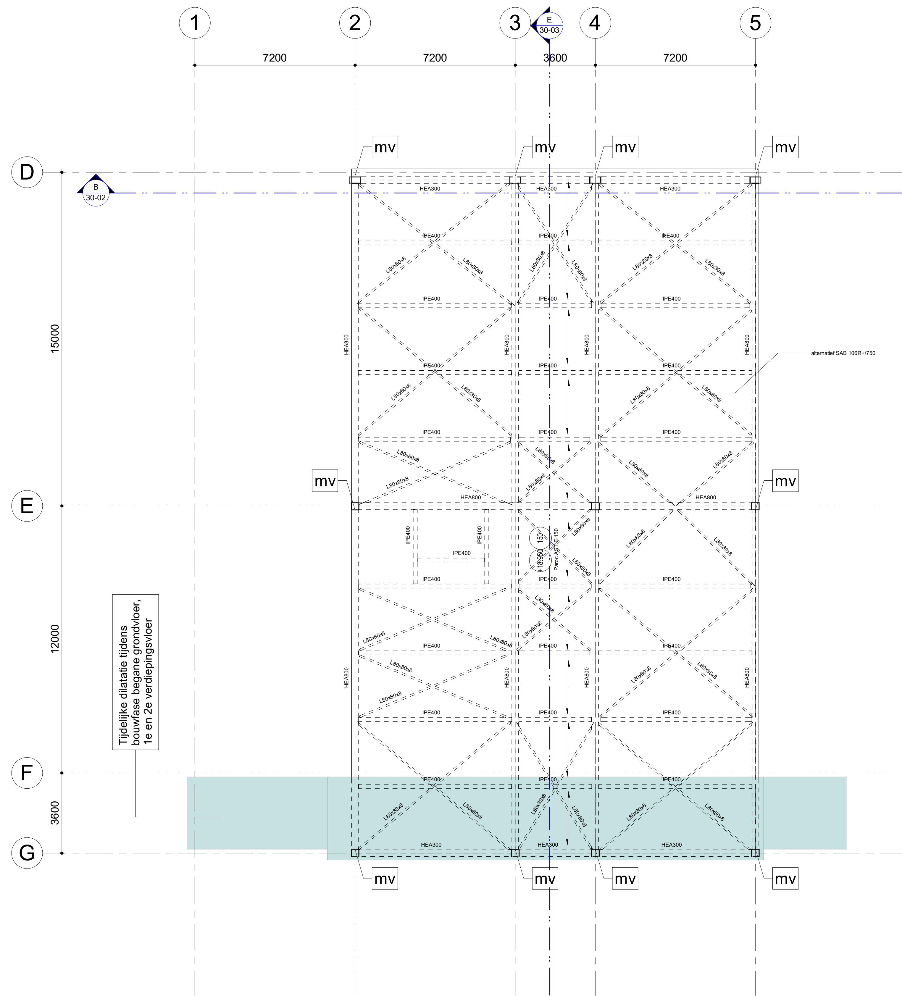
1 Dak B Schaal: 1:100
