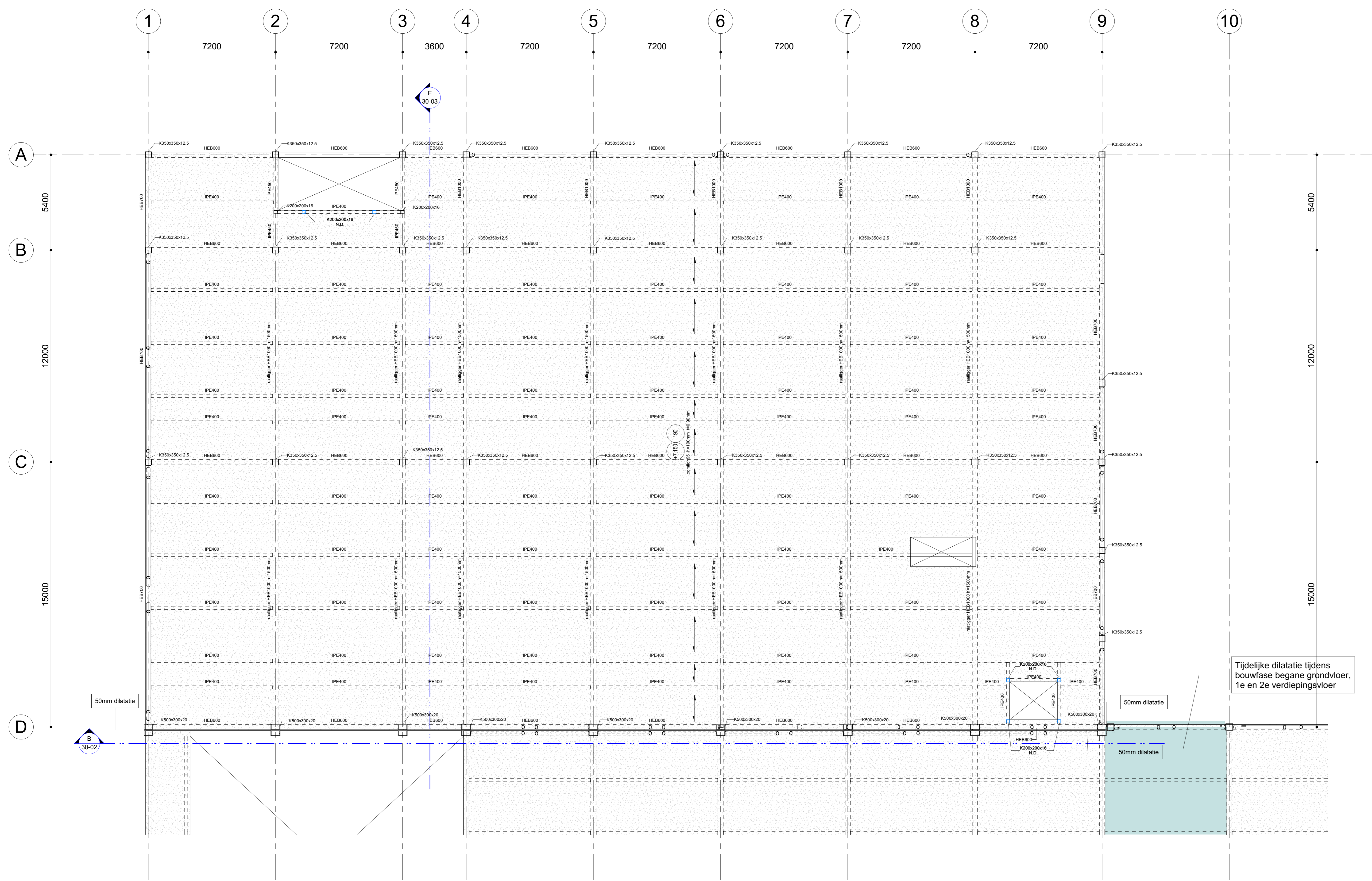
1 1e verdieping Schaal: 1:100
