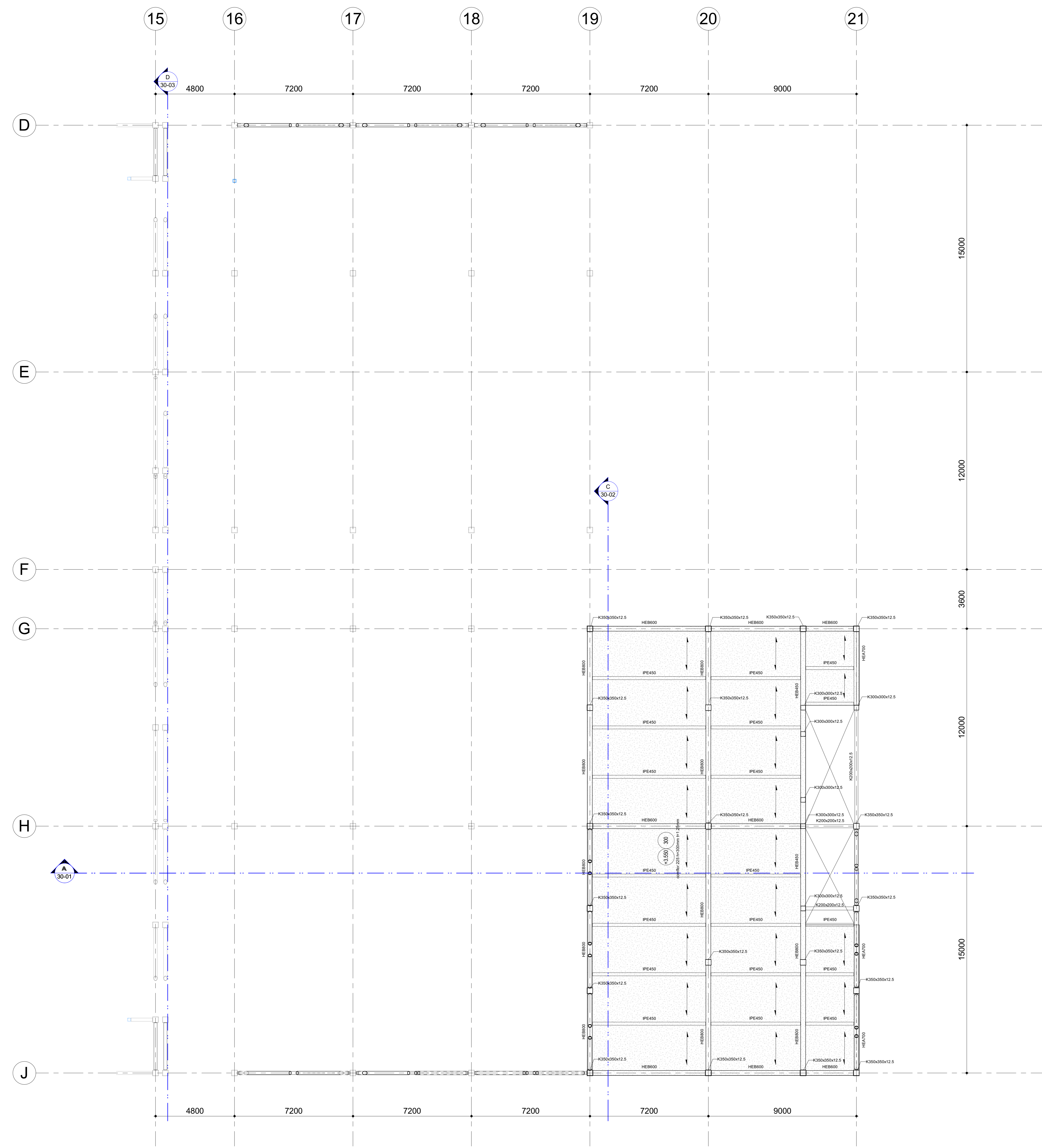
1 MEZZANINE Schaal: 1:100
