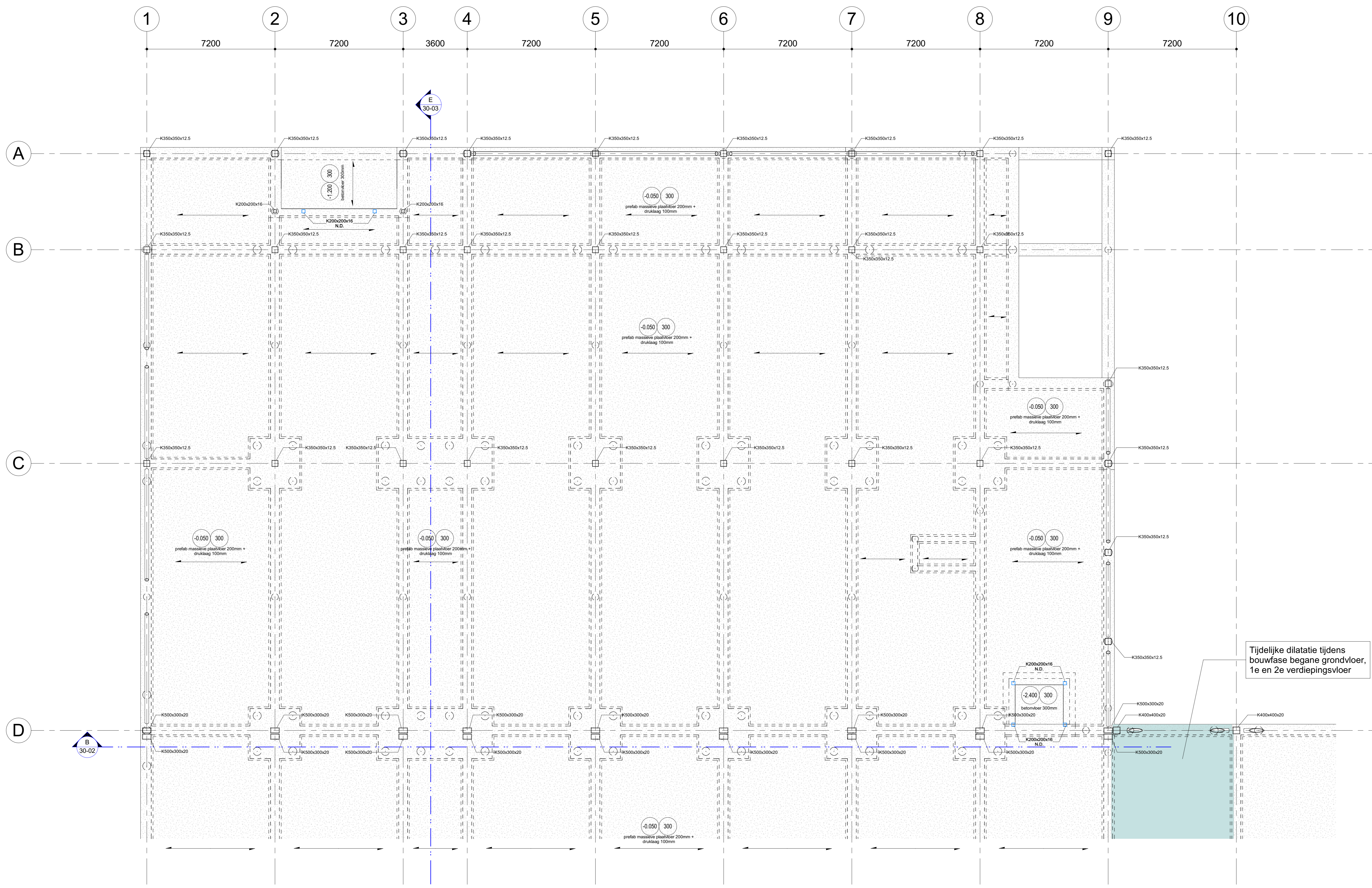
1 Begane grondvloer Schaal: 1:100
