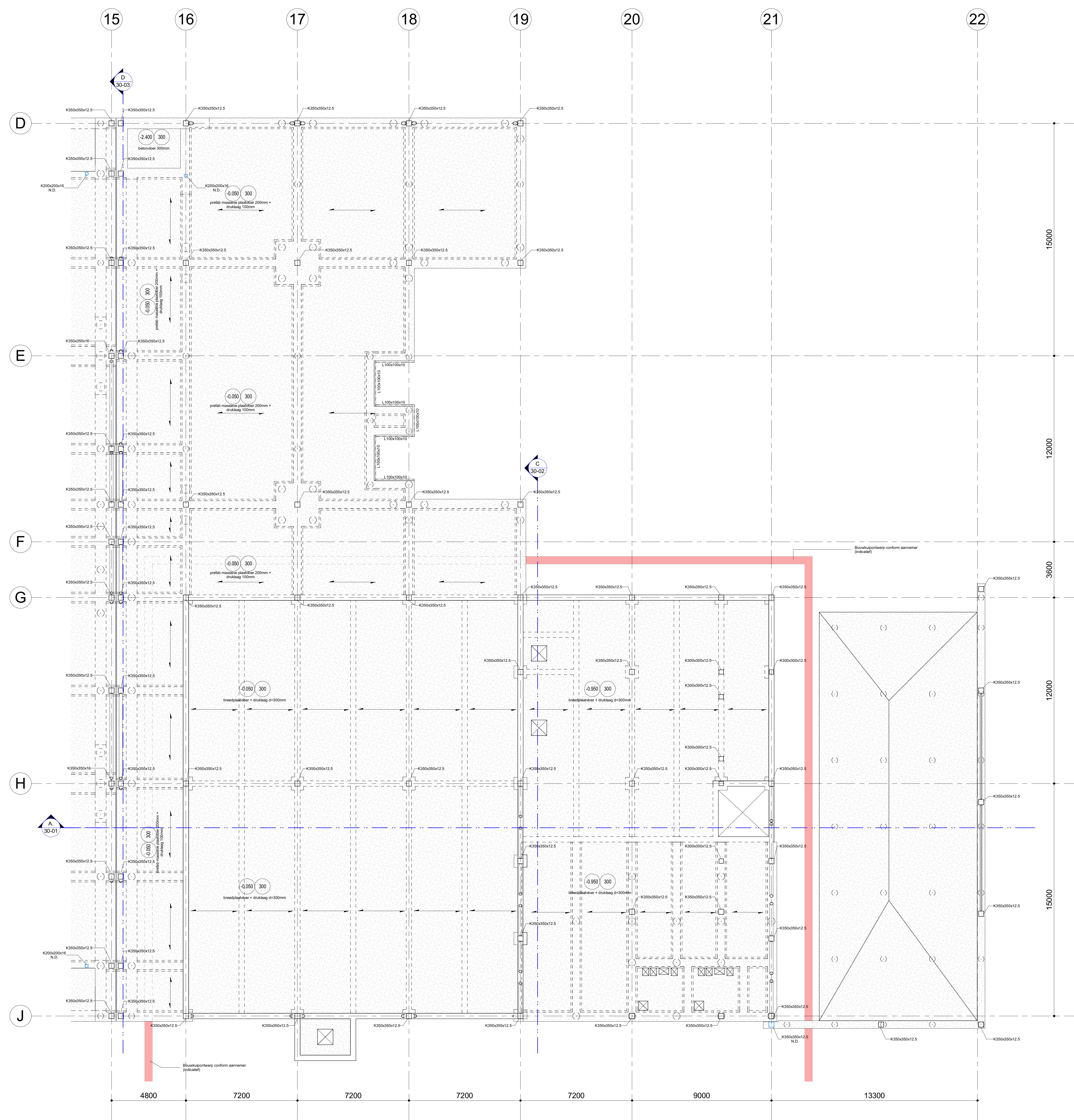
1 Begane grondvloer Schaal: 1:100
