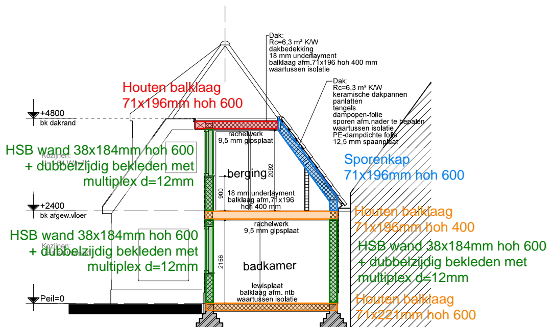
DOORSNEDE A-A
