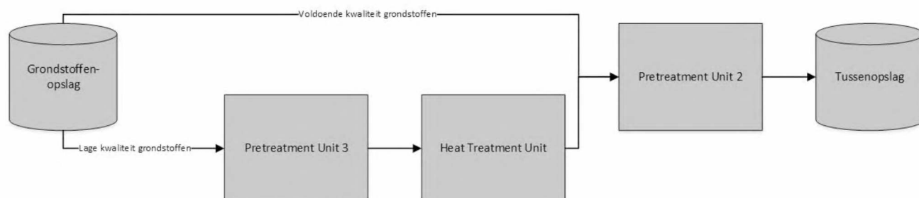
Figuur 3-2: Schematisch overzicht van de NExPRE-unit
