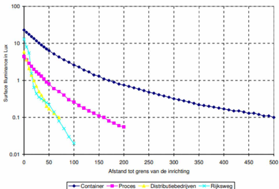
Figuur 2 Directe lichtinval als functie van de afstand tot de inrichting (Bron Figuur: figuur 4.3 uit ZE 2007 ).
