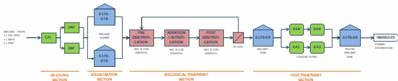
Figuur 2.2: Block flow diagram hoofdproces AWZI
