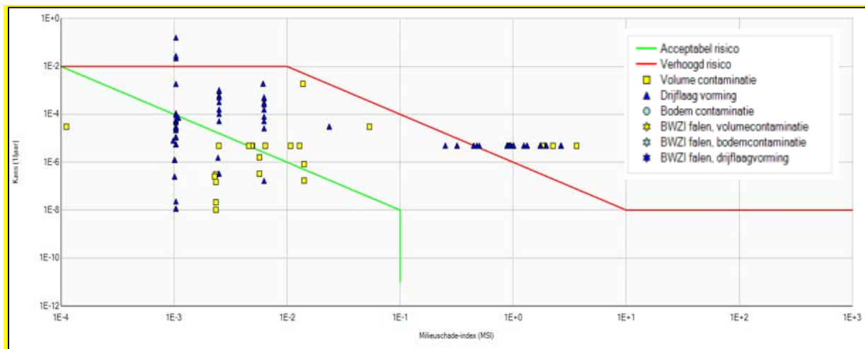
Figuur 0.3: MSI-grafiek [3]
