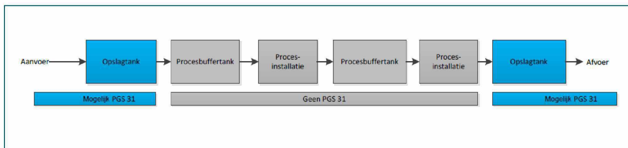
Figuur 1: Schematische weergave verschil opslagtank en processtank
