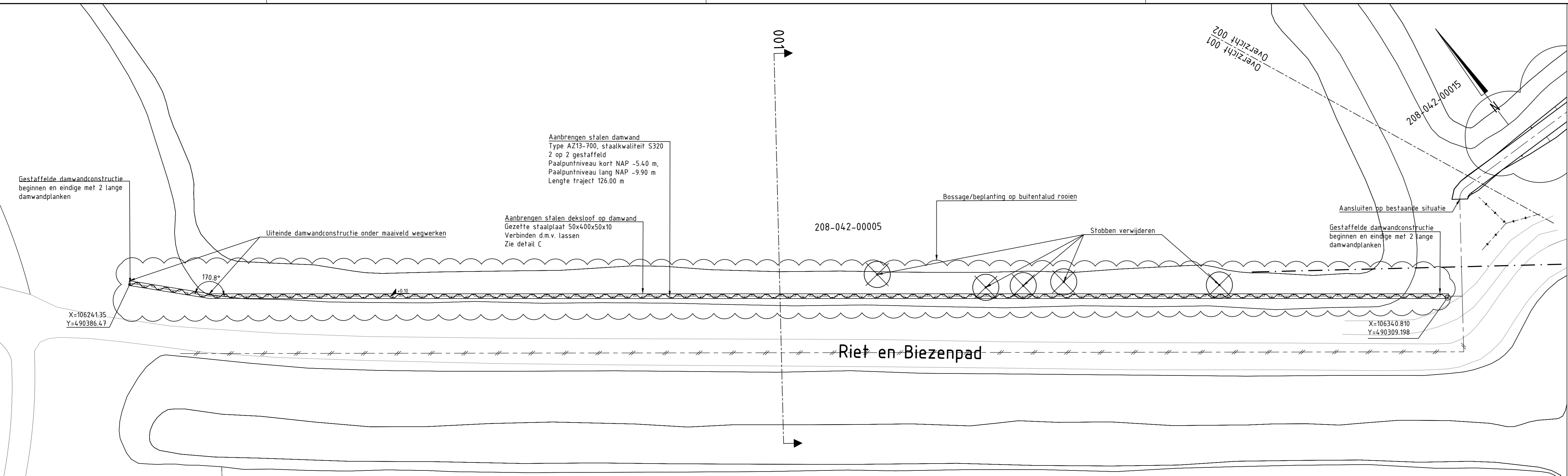
OVERZICHT 001 Schaal 1:200
