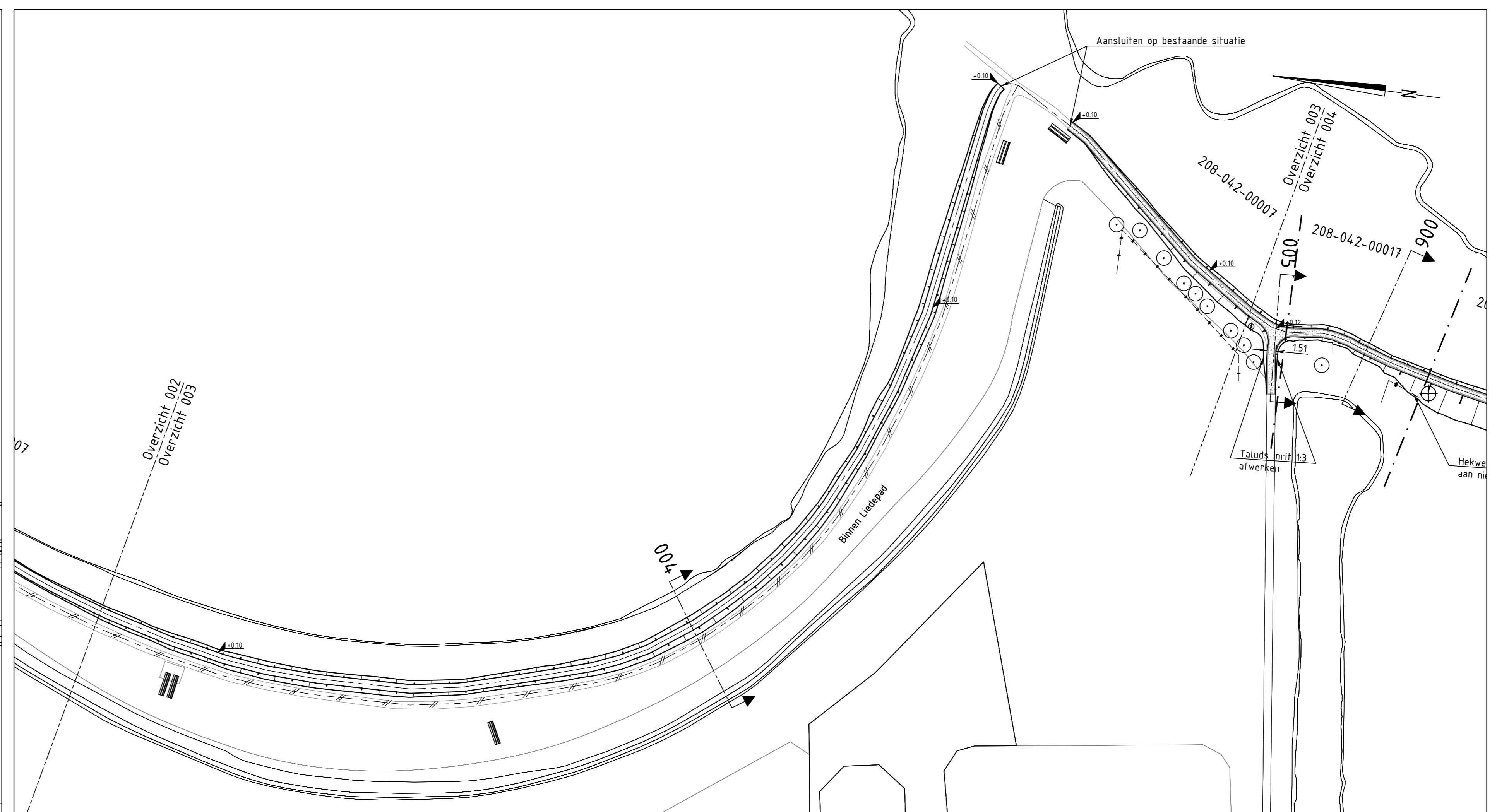
OVERZICHT 003 Schaal 1:500
