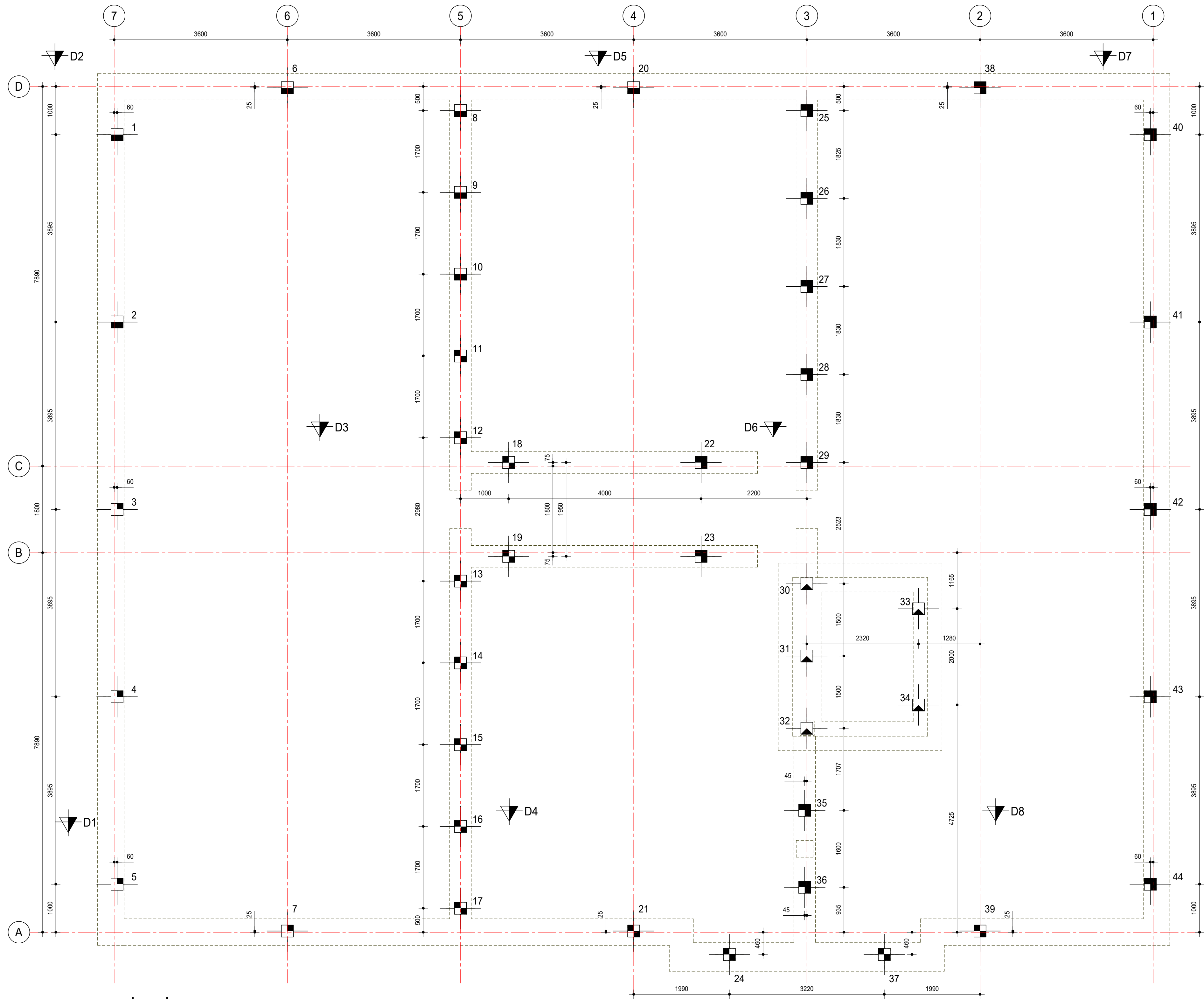
palenplan
