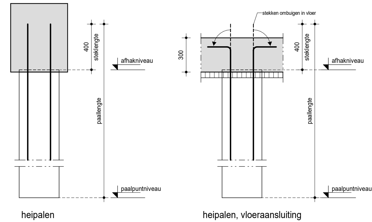
paalaansluiting principe
